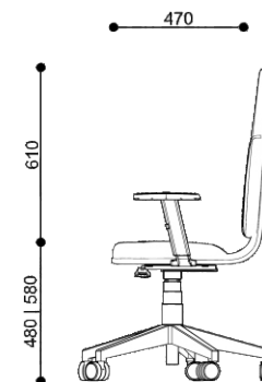
Cadeira New Top G / Medida em milímetros
