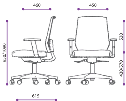
Cadeira Shape / Medida em milímetros
