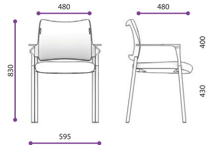
Cadeira Task / Medida em milímetros
