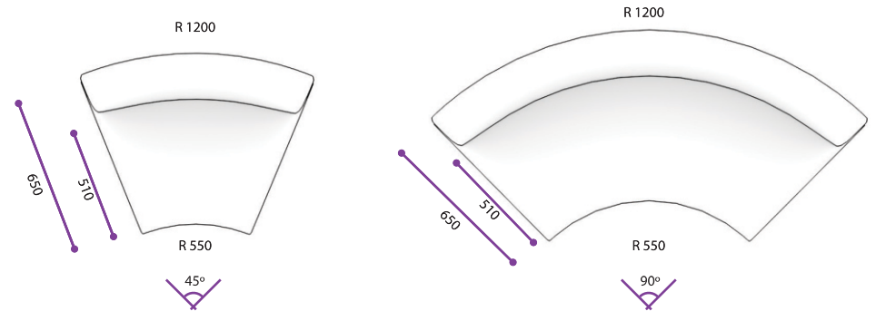
Sofá Mod / Medida em milímetros
