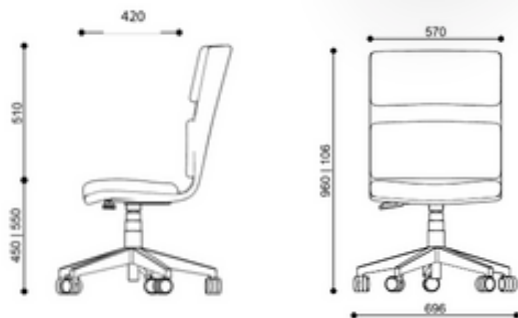
Cadeira Easy Média / Medida em milímetros
